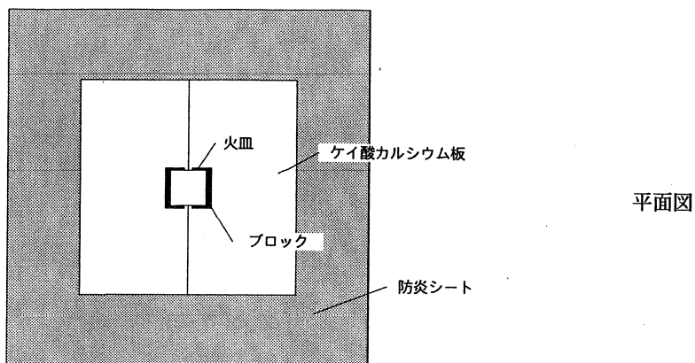
火皿配置方法
