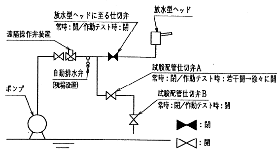
遠隔操作弁装置周り（作動テスト時）
