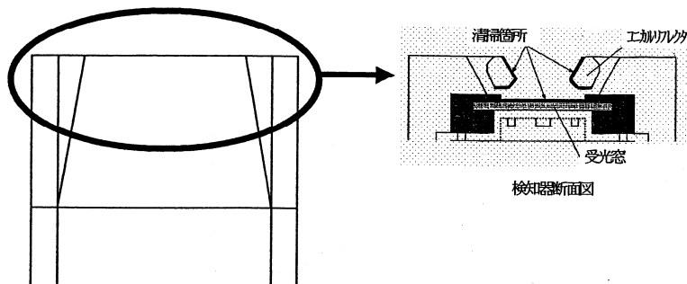
炎検知器の清掃箇所
