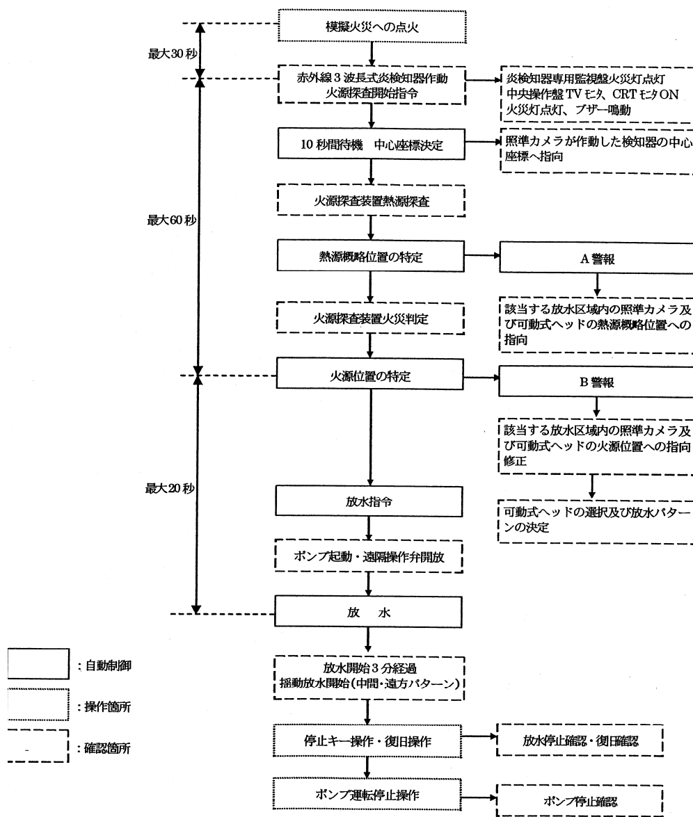
総合点検フロー図
